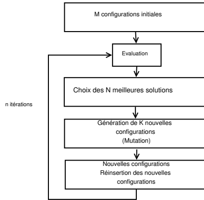
FIG. 1 – Algorithme d'optimisation
