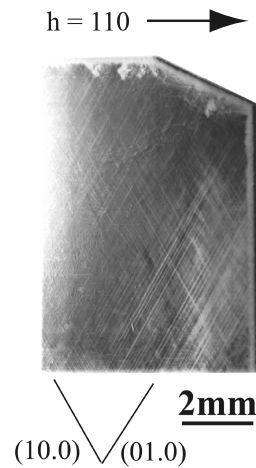
Fig.4 Topographie en transmission du film Zn 0.9 Mn 0.1 O (400nm) : réflexion 110, radiation Mo K \alpha_1 .
