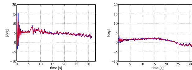
(e) Roll angle \varphi(t) : roll angle command (red), actual angle (blue).
