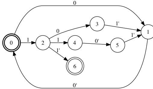
FIGURE 13. Automate \mathcal{A}_{L^{\text{rat}}} de l'exemple 3.17
