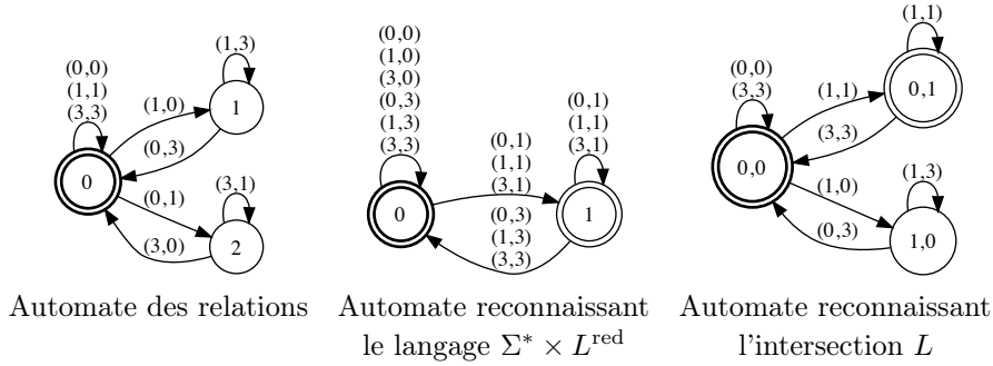
FIGURE 14. Construction d'un automate reconnaissant le langage L de la preuve ci-dessus pour l'exemple 3.14
