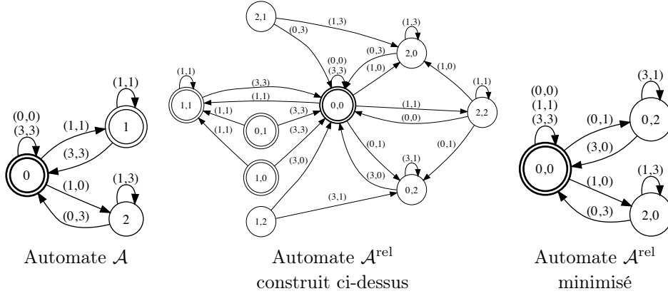
FIGURE 15. Construction d'un automate reconnaissant le langage L^{\text{rel}} à partir d'un automate reconnaissant le langage L = L^{\text{rel}} \cap (\Sigma^* \times L^{\text{red}}) pour l'exemple 3.14
