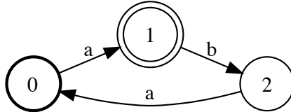
FIGURE 7. Automate reconnaissant l'ensemble des mots de la forme a(baa)^n .
