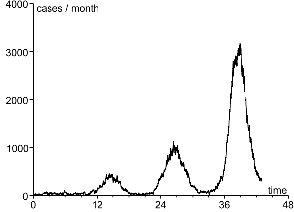
FIGURE 2 – Nombre de cas rapportés c\tilde{I}(t) en fonction du temps (en mois) dans une simulation du processus de naissance et de mort en utilisant les valeurs de paramètres (17). La condition initiale est \tilde{E}(t^*) = 3 et \tilde{I}(t^*) = 2 .
