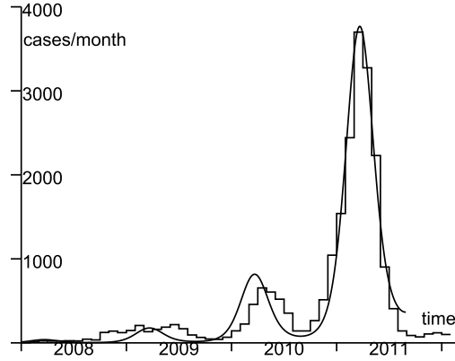
FIGURE 1 – Nombre mensuel de cas de rougeoles rapportés (fonction en escalier) de janvier 2008 à février 2012 (données de InVS (2012) et Parent du Châtelet et al. (2010)). Meilleur ajustement (courbe lisse) aux données de janvier 2008 à juillet 2011.
