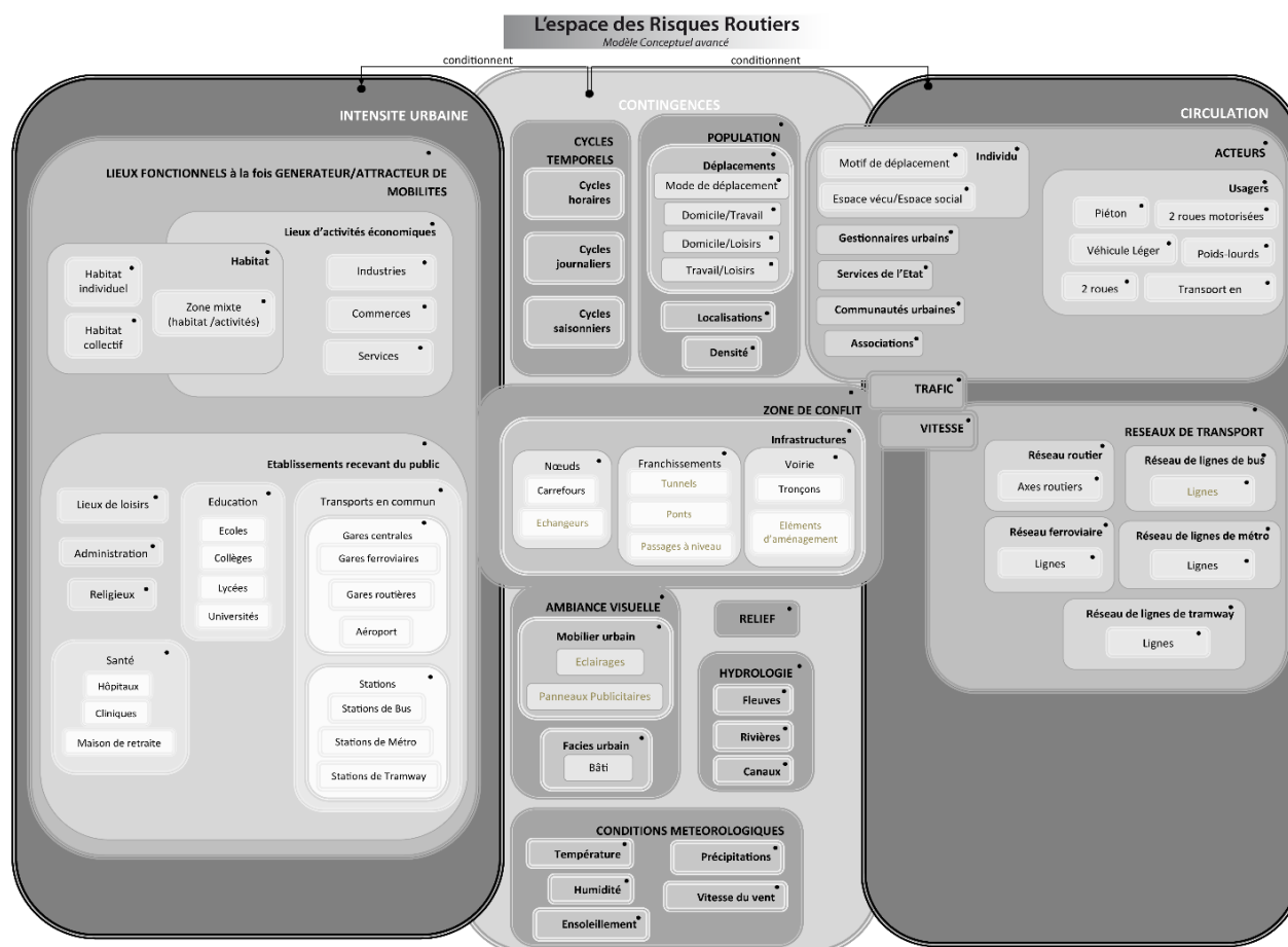
Figure 6 : Modèle Conceptuel de Données du projet CRITERE
