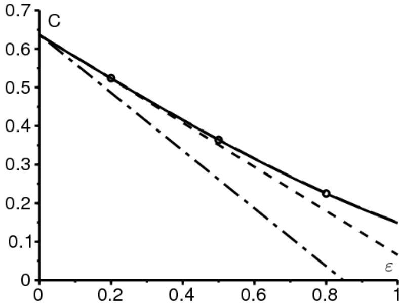
图2.中频：使用杂环曲线[实线]或偏微分方程[长虚线]（两条线几乎无法区分）计算的数 C ，浮点乘数如图1 [点]，近似公式 (19) [短虚线]和低频公式 (20) [长虚线]，具体取决于 \varepsilon 。与图1相同的参数值
