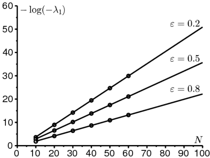
图1.主方程的Floquet乘数的计算： -\log(-\lambda_1) 作为一个功能 \tilde{N} 为 \varepsilon \in \{0,2; 0,5; 0,8\} 和 N = 10, 20, \dots, 60 。数字 C 是这些线的斜率。参数值： T = 1, a_0 = 20, b = 5 。
