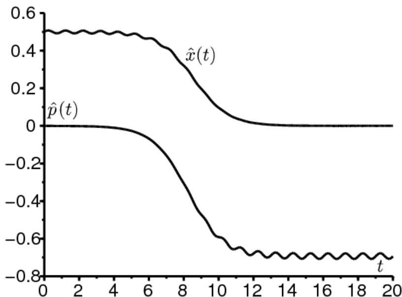
图5.组件 t \mapsto \hat{x}(t) 和 t \mapsto \hat{p}(t) 两个周期解的杂散轨道的变化 (0, p^*(t)) 和 (x^*(t), 0) 。与图4中相同的参数值和 \varepsilon = 0,1 。
