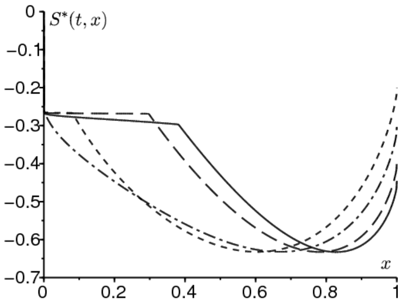
图3.定期解决方案 S^*(t, x) 哈密顿-雅可比方程，绘制成的函数的 x 为 t = 0 （实线）， t = T/4 （长虚线）， t = T/2 （短虚线）和 t = 3T/4 （长短虚线）。参数值与图1和 \varepsilon = 0,5 。
