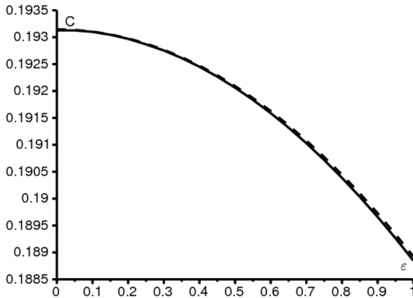
图4.高频状态： C 是根据 \varepsilon 的函数，使用杂环曲线[实线]和高频公式 (22) [虚线]计算的。参数值： T = 1 , a_0 = 2 , b = 1 。
