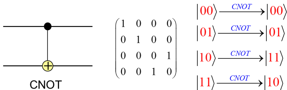
Figure 4. Porte quantique unitaire et réversible CNOT pour deux qubits.
