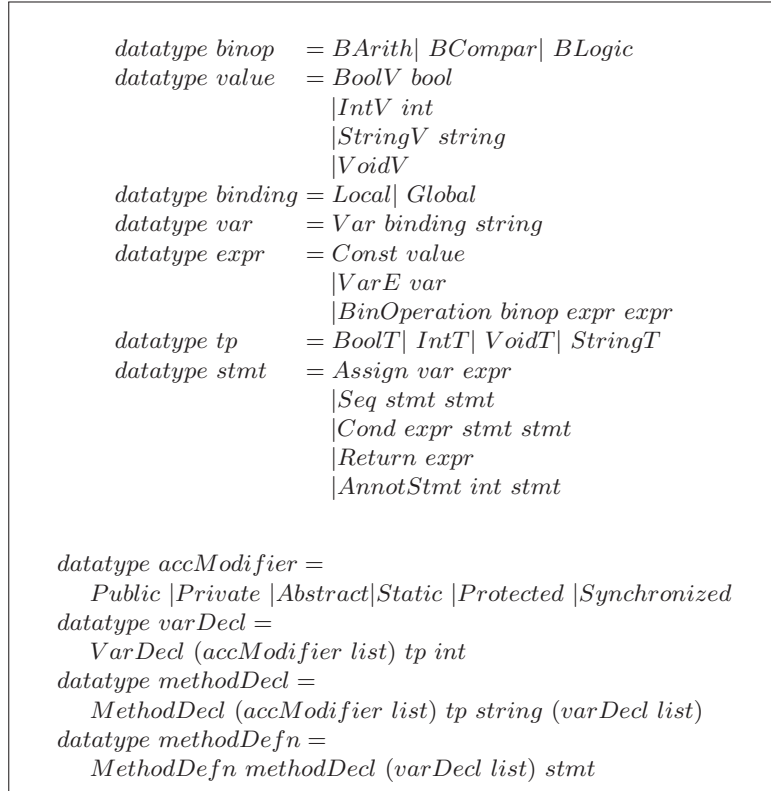
Fig. 6. Datatypes in Isabelle
