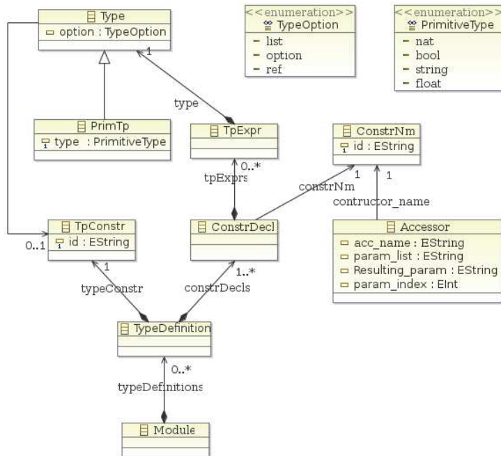
Fig. 3. Datatype Meta-model
