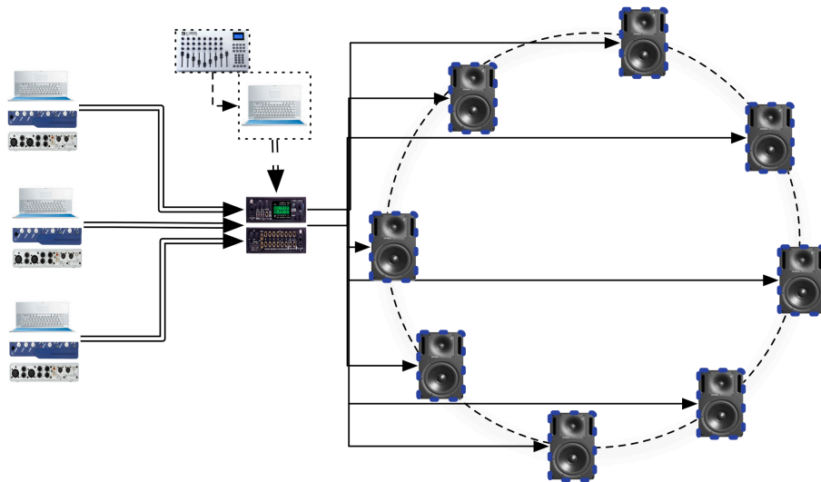
Figure 5 : schéma de routage du signal et contrôle de la distribution spatiale.
