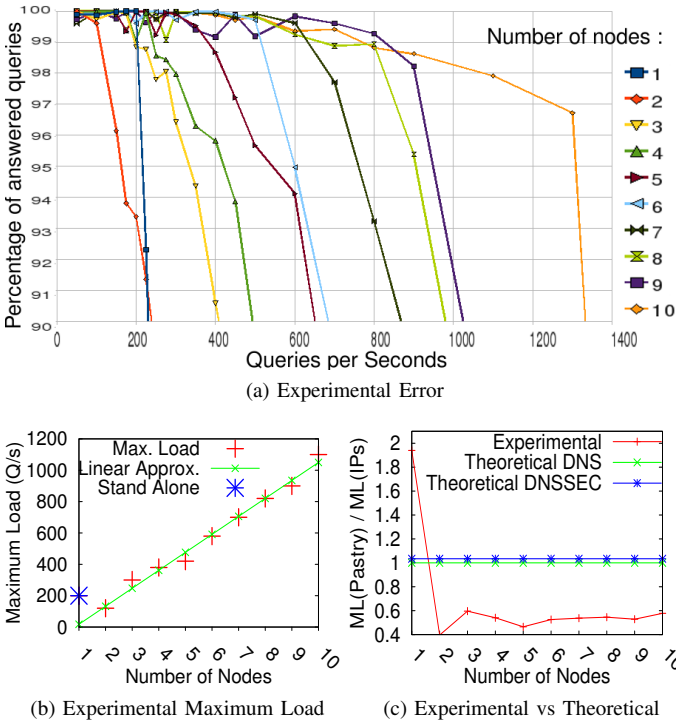
Fig. 8. Maximum Load
