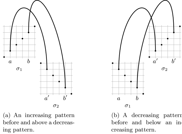
Fig. 2. Illustration of Lemma 3.
