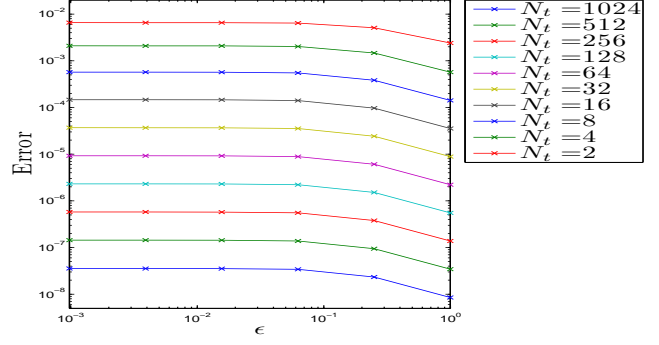
(b) err_{(S^\epsilon, A^\epsilon)}(T_f = 0.2) w.r.t \epsilon , N_x = 2^8
