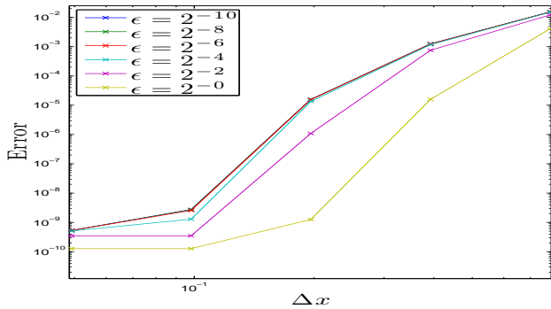
(a) err_{(S^\varepsilon, A^\varepsilon)}(T_f = 0.2) w.r.t \Delta x , N_t = 2^{15}
