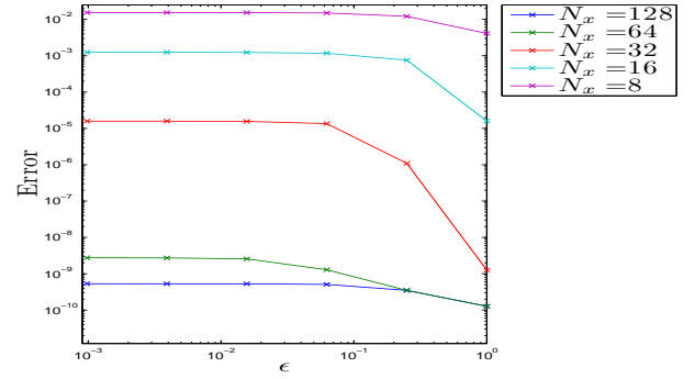
(b) err_{(S^\epsilon, A^\epsilon)}(T_f = 0.2) w.r.t \epsilon , N_t = 2^{15}
