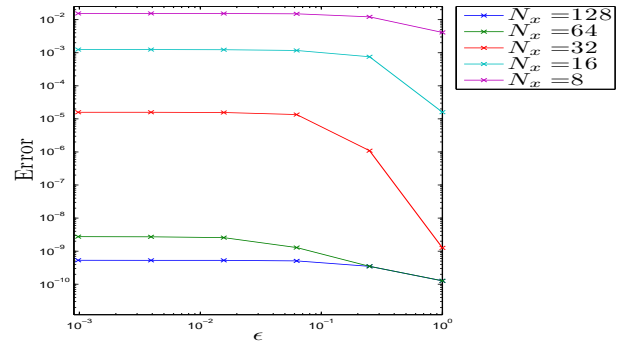
(b) err_{(S^\varepsilon, A^\varepsilon)}(T_f = 0.2) w.r.t \varepsilon , N_t = 2^{15}
