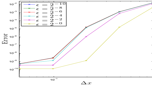
(a) err_{(S^\epsilon, A^\epsilon)}(T_f = 0.2) w.r.t \Delta x , N_t = 2^{15}
