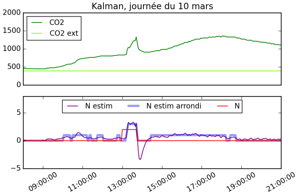
Figure 16 : Comportement du filtre de Kalman lors de variations de C_{ext}
