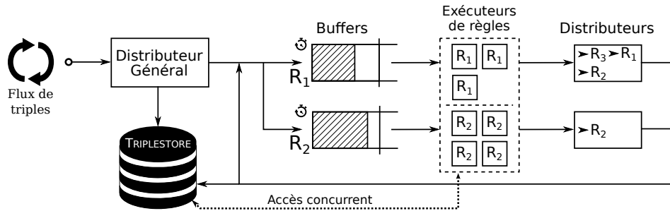
FIG. 1 – Vue d'ensemble de l'architecture du raisonneur Slider
