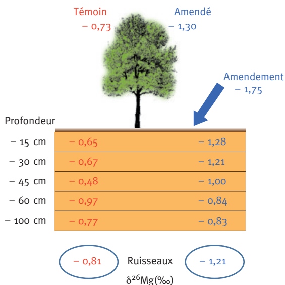
FIGURE 1 COMPOSITION ISOTOPIQUE EN Mg MESURÉE DANS LES SOLS, LES EAUX ET LES ARBRES (HÊTRES) DES BVF DE CORNIMONT, SUR GRANITE, 7 ANS APRÈS L'APPORT. À gauche, BVF témoin, à droite BVF amendé (d'après Bolou-Bi et al. , soumis)
