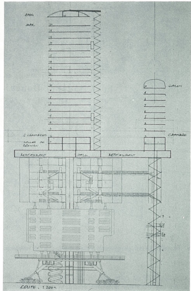
● Hérouville Saint-Clair, la Tour Européenne. Coupe. Photo: Ville d'Hérouville Saint-Clair
