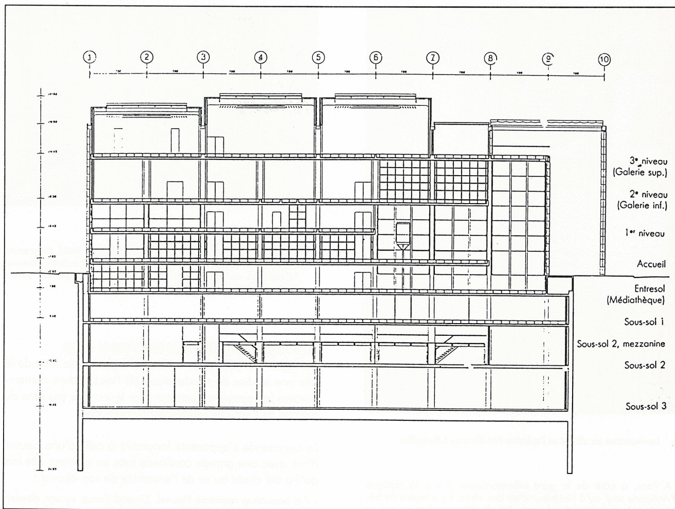
● La médiathèque à Nîmes, coupe.
