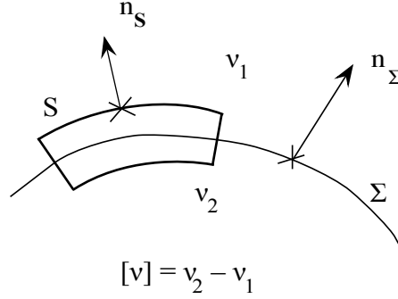
Figure 1: (Le saut [\nu] d'une quantité scalaire telle que \nu au passage d'une interface matérielle telle que \Sigma est sa valeur 'en amont' moins sa valeur 'en aval' du flot imaginaire traversant \Sigma dans le sens de la normale n_\Sigma . Ici, avec \nu constant de part et d'autre de \Sigma , on a donc [\nu] = \nu_2 - \nu_1 .) L'intégration de {}^M T \cdot n_S sur la surface S donne la force magnétique exercée sur la partie de \Sigma intérieure à S . On retrouve de cette façon, et plus simplement, le résultat obtenu en interprétant l'expression \frac{1}{2} |B|^2 \nabla \nu du champ de forces [2] au sens des distributions, soit \frac{1}{2} (|H_\tau|^2 [\mu] - B_n^2 [\nu]) n_\Sigma , où H_\tau et B_n sont les composantes tangentielle de H et normale de B au droit de \Sigma (cf. [2]).
