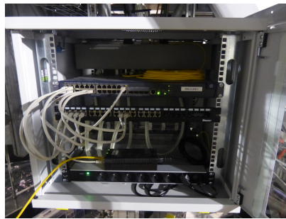
(b) Commutateur placé sur la plaque relié via un transceiver 10Gb/s bidi (simplex)
