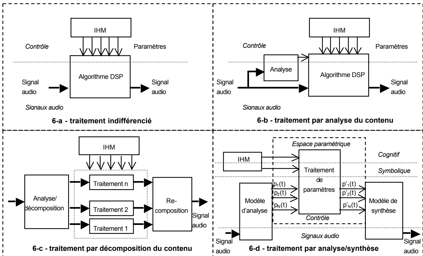
FIG. 6 : Structures de traitement et de contrôle
