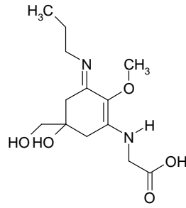
Asterina-330
