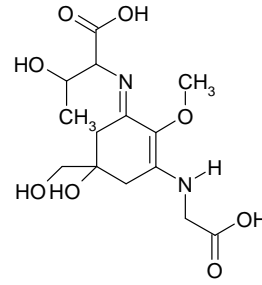
Porphyra-334
