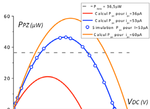
fig.12. Puissance fournie par le récupérateur P_{PZ} vs V_{DC} .
