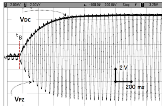
fig.8 Evolution de V_{PZ}(t) et de V_{DC}(t) .
