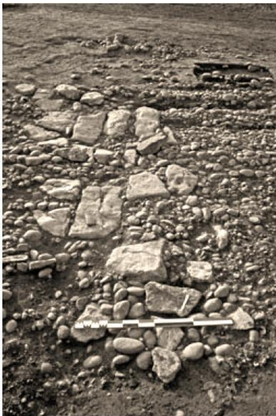
Fig. 14 : Détail de l'empièrrement d'une des voies (V2) du Parc de l'Aéroport, à Pérols, renforcé à l'emplacement d'un fossé de l'âge du Fer.
