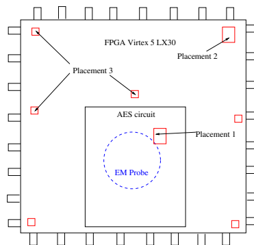
Fig. 9: Platform EM Measurement
