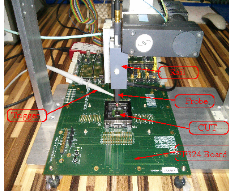
Fig. 8: Platform EM Measurement
