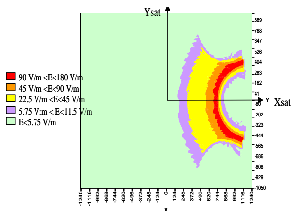
Figure 1. La cartographie du champ électrique (valeurs maximales) sur les panneaux terre d'un satellite géostationnaire ( f=17.7\text{GHz} , puissance rayonnée 70 W).
