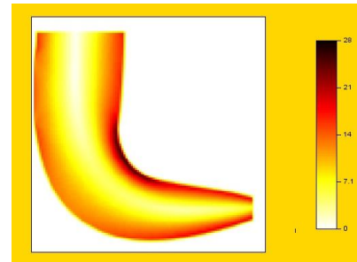
Fig 12: von Mises level
