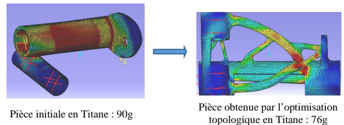
Figure 4. RESULTATS DU CALCUL ELEMENTS FINIS
