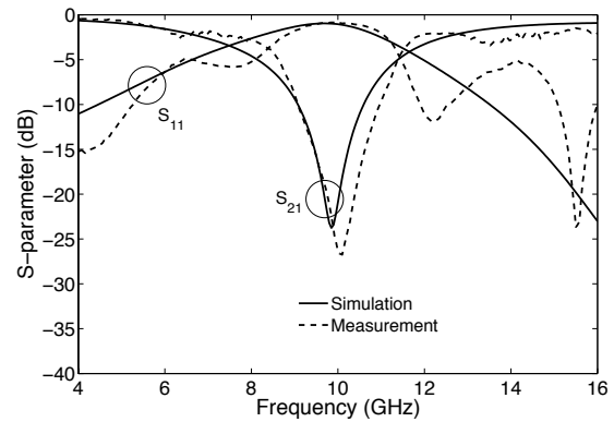
Figure 7. Simulation et mesure du filtre large bande et coupe-bande d'ordre 1. La bande passante relative mesurée à 10 dB est BW_{10dB} = 18\% .
