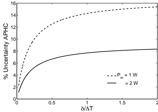
Figure 9. Incertitude en % sur la mesure d'APHC en fonction de \delta/\Delta T , de la puissance P_{in} . Dans cet exemple \delta = 1\text{ }^\circ\text{C} , T_{amb} = 22\text{ }^\circ\text{C} et T_{ref} = 28\text{ (33)}\text{ }^\circ\text{C} pour P_{in} = 1\text{ (2)}\text{ W} , respectivement.
