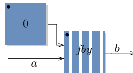
FIGURE 11 – Bloc mem de FAUST
