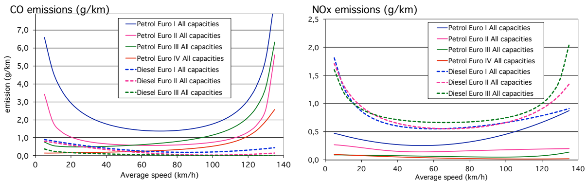
Figure 7 : Courbes d'émission types de la méthode Copert4 : CO et NOx (tous types de voitures essence et diesel)
