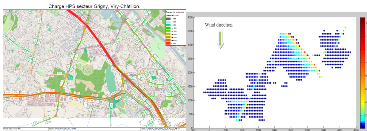
Figure 6 - Configuration de simulation du trafic, et de la pollution atmosphérique (CopCete, Polyphemus) et des eaux (SWMMM) en métaux Cd, Zn, et Pb, sur la zone expérimentale de Grigny. A droite, concentrations de zinc ( \text{ng}/\text{m}^3 ) dues au trafic.
