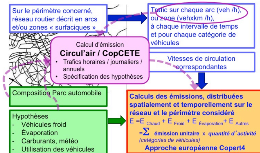
Figure 10 : Étape de calcul des émissions de polluants à partir de la modélisation des déplacements et trafics sur le réseau routier modélisé (projet ANR Eval-PDU)
