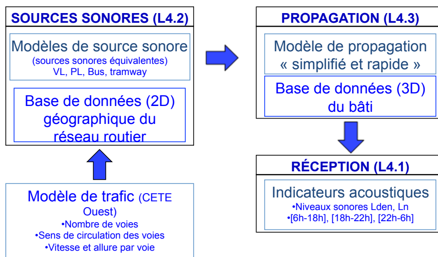
Figure 12 : Démarche générale de simulation des niveaux de bruits à partir de la modélisation des déplacements et trafics sur le réseau routier modélisé (projet ANR Eval-PDU)
