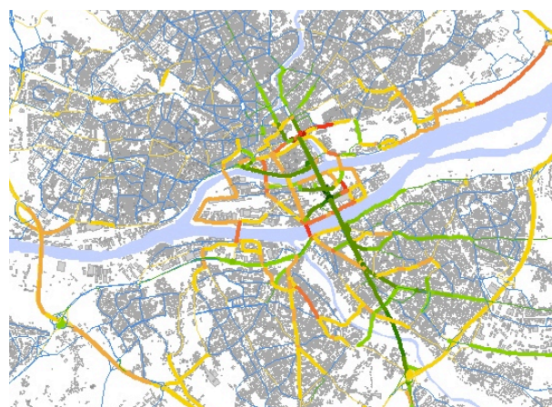
Figure 2. Évolution de l'émission de NOx (réf. 2008)
