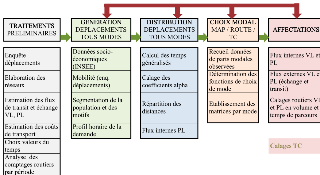
Figure 9 : Approche de la modélisation des déplacements et trafics (modèle VISEM - VISUM), utilisée dans le projet ANR Eval-PDU
