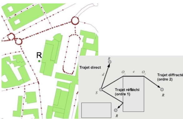
Figure 13 : Décomposition du trafic en points sources acoustiquement homogènes et propagations directes, réfléchies, diffractées
