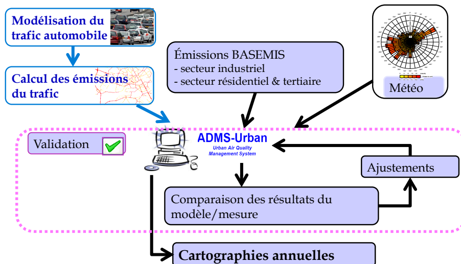
Figure 11 : Du trafic aux concentrations de polluants, avec prise en compte des autres sources, de la météo, et avec ajustements aux observations des stations de mesure de la qualité de l'air (projet ANR Eval-PDU)
