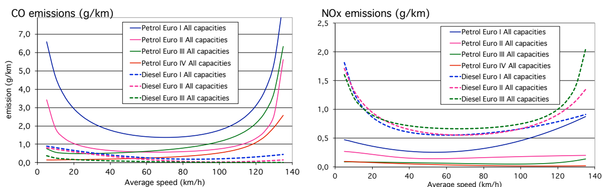
Figure 7 : Courbes d'émission types de la méthode Copert4 : CO et NOx (tous types de voitures essence et diesel)
