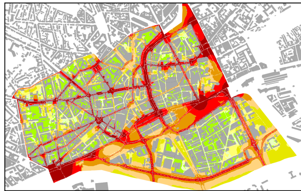
Figure 14 : Modélisation simplifiée 2D et production de carte de bruit dans OrbisGIS
