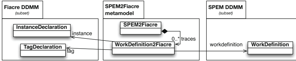
Fig. 5. SPeM2Fiacre trace metamodel
