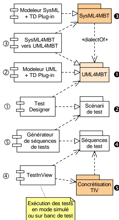
Figure 1 : Génération de séquences de test à partir de modèles SysML
