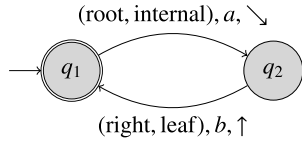
Fig. 2. A deterministic tree walking automaton.
