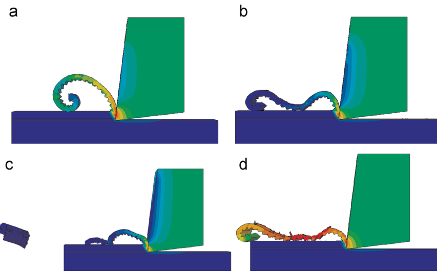
Fig. 13. Temperature field: (a) Conventional lubrication, (b) P=50 bar, (c) P=100 bar, (d) P=100 bar ( h=0 ).
