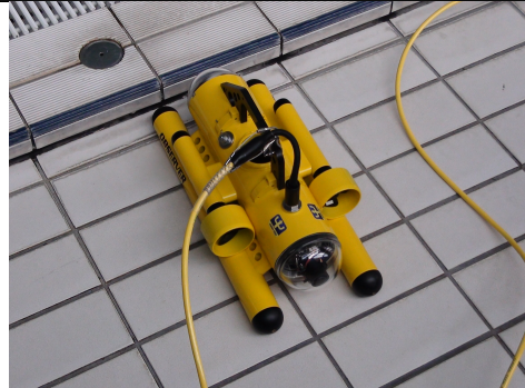
Mini-ROV téléopérable par Internet (extrait de EVR@-WE, projet européen FP7 DIGITAL OCEAN EU )
