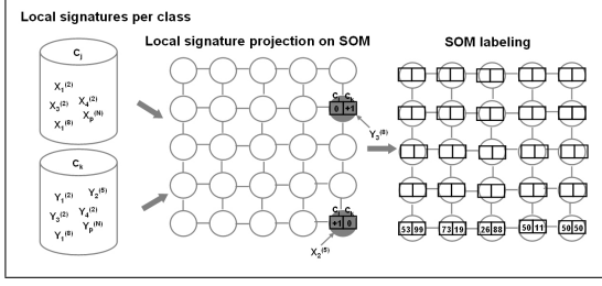
Figure 3. SOM labeling.
