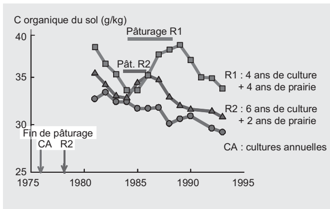
FIGURE 1 : Effet à long terme des cultures annuelles et de 2 rotations cultures annuelles - prairie sur les teneurs en C organique dans un essai de longue durée en Argentine (d'après STUDDERT et al. , 1997). FIGURE 1 : Long-term effects of annual crops and 2 ley- arable rotations on organic C levels in a long-term experiment in Argentina (after STUDDERT et al. , 1997).
