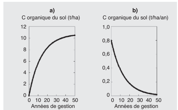
FIGURE 2 : Evolution de l'accumulation du carbone organique (a) et taux annuel d'accumulation de C (b) sous prairie (d'après FRANZLUEBBERS et al. , 2012). FIGURE 2 : Changes in the accumulation of organic C (a) and the annual rate of C accumulation (b) in pastures (after FRANZLUEBBERS et al. , 2012).
