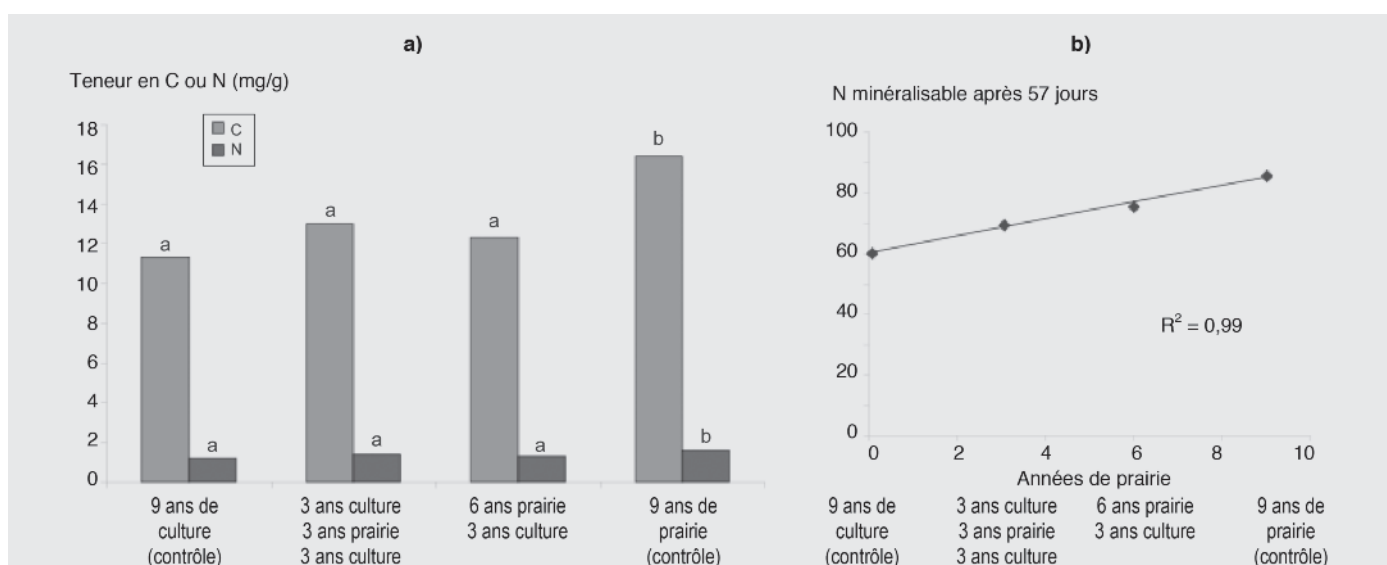
FIGURE 4 : Evolution de la teneur des sols du SOERE ACBB (site de Lusignan) en C et N (a) et en N minéral potentiellement minéralisable (b) après 9 années de traitements.
