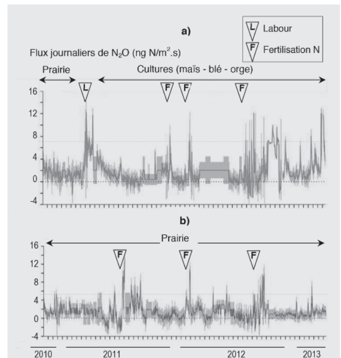
FIGURE 6 : Flux journaliers de N_2O pour a) une rotation prairie - cultures et b) une prairie continue.
