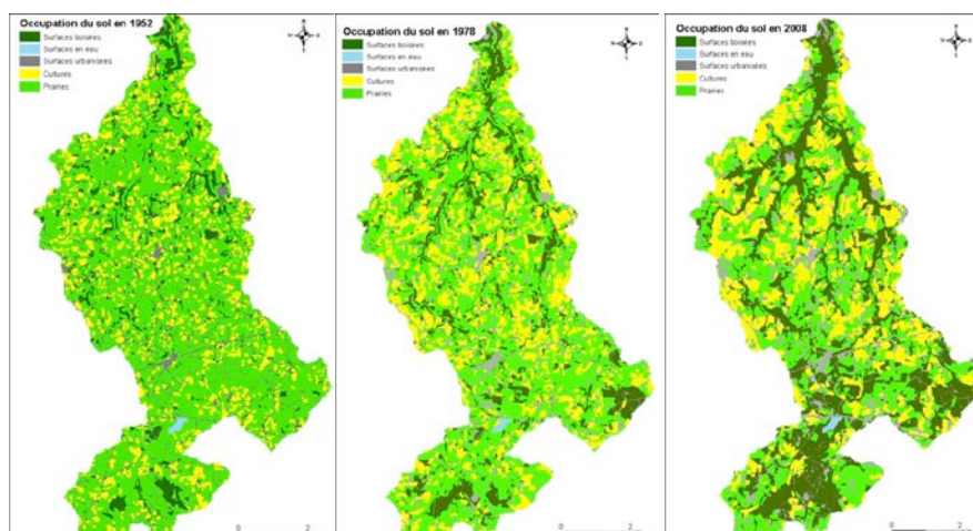
Figure 5 : Evolution de l'occupation des sols du bassin versant du Yar de 1950 à nos jours (à partir de photos aériennes et de données satellites)
