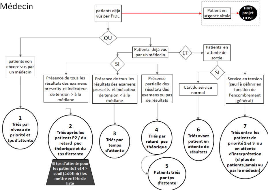
Figure 2. Algorithme de tri médecin
