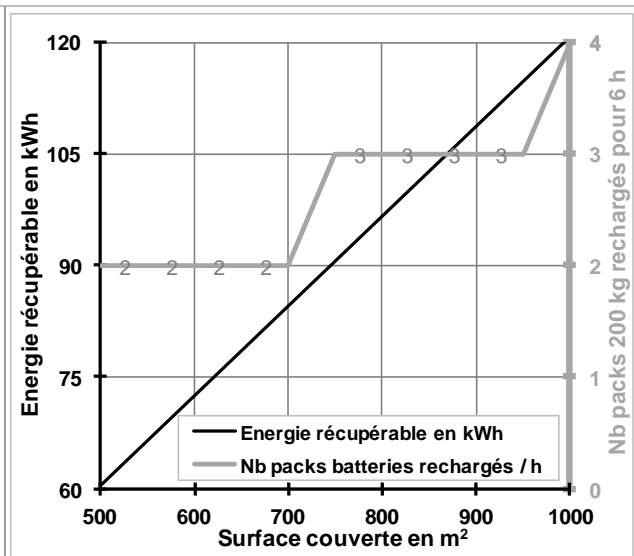
Fig. 9 – Énergie récupérable en kWh (ordonnée de gauche) et nombre de packs de batteries (ordonnée de droite) pouvant être rechargés en 6 heures d'ensoleillement en fonction de la surface de hangar couverte par des panneaux photovoltaïques.
