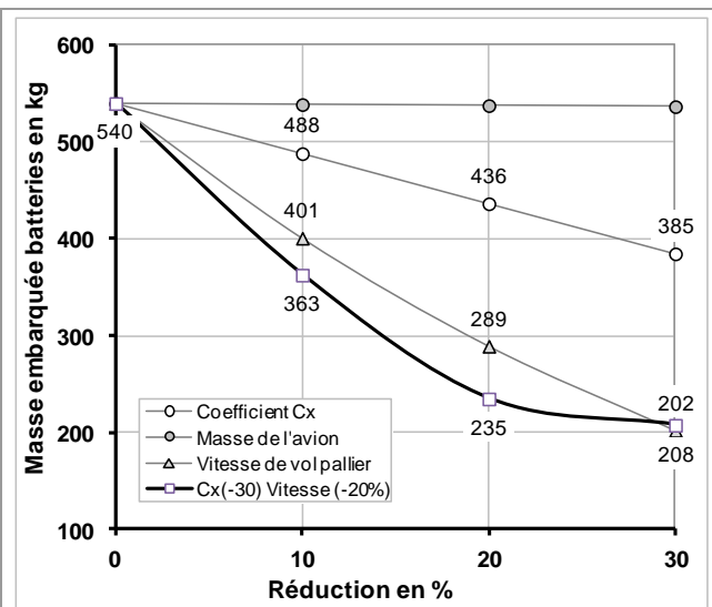
Fig. 7 – Évolutions de la masse embarquée de batteries en fonction du pourcentage de réduction pour le coefficient C_x , la vitesse de croisière et la masse de l'avion. Pour la courbe noire, la réduction de la vitesse de vol est limitée à 20%.
