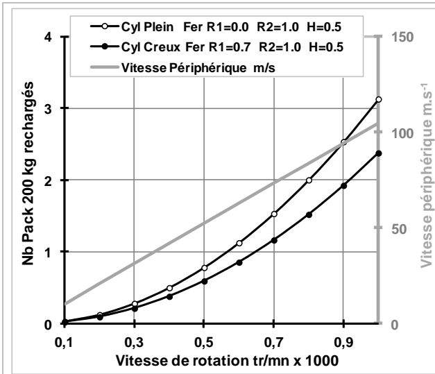
Fig. 12 – Nombre de packs de batteries (ordonnée de gauche) pouvant être rechargés par des volants d'inertie, cylindres plein et creux, en fonction de la vitesse de rotation en tr/mn. Les vitesses périphériques sont reportées sur l'ordonnée de droite.
