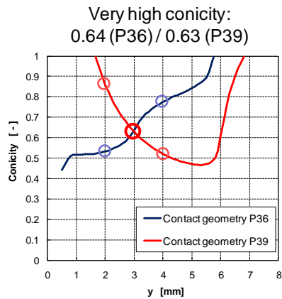
Fig. 10: Conicity of contacts P36 et P39.
