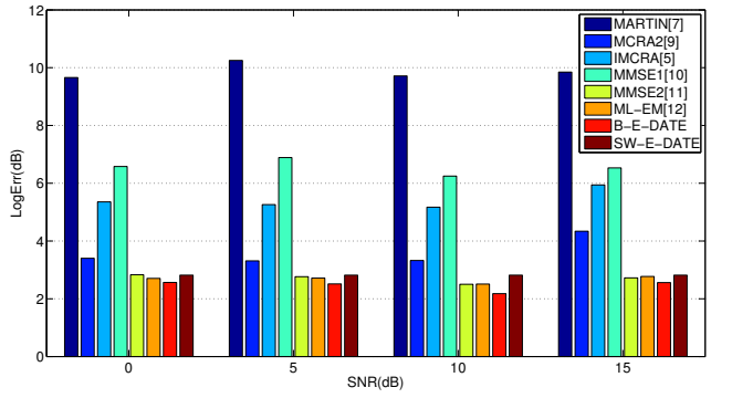
(d) train noise
