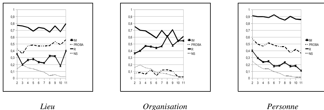
Diagramme 1 à 3 : F-mesure pour les Lieux, les Organisations et les Personnes.
