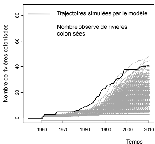
Figure 50: Prédiction issue du modèle à partir d'un scénario fictif ne comprenant qu'une seule introduction en 1962 dans la Rivière du Château. On peut observer que la majorité des trajectoires simulées est bien en dessous de la dynamique réelle, avec un nombre de rivières colonisées bien inférieur au final. Cette simulation est une illustration du rôle des introductions multiples sur le plan démographique.
