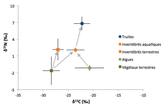
Figure 47: Résultats des analyses isotopiques sur carbone ( \delta^{13}\text{C} ) et azote ( \delta^{15}\text{N} ) réalisées à partir des échantillons biologiques prélevés à Kerguelen. Les producteurs primaires (en vert) et consommateurs primaires (en orange) ont été collectés sur les cours d'eau (ronds) ou leurs berges (carrés). En haut du réseau trophique, les truites figurent en bleu. Des flèches grises représentent le fractionnement trophique ; dans le cas des invertébrés aquatiques la contribution de 2 sources de carbone en mélange (aquatique et terrestre) est indiquée.
