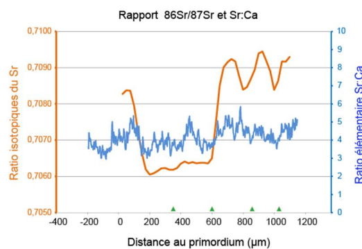
Figure 26: Profils microchimique (bleu) et isotopique (orange) d'un poisson. La signature microchimique fluctue autour d'une valeur intermédiaire et ne permet pas de déterminer avec certitude l'utilisation de l'habitat. En revanche, la signature isotopique révèle une ascendance marine, suivie d'une période de croissance juvénile en milieu dulçaquicole et d'un passage rapide en milieu marin, sans période transitoire.
