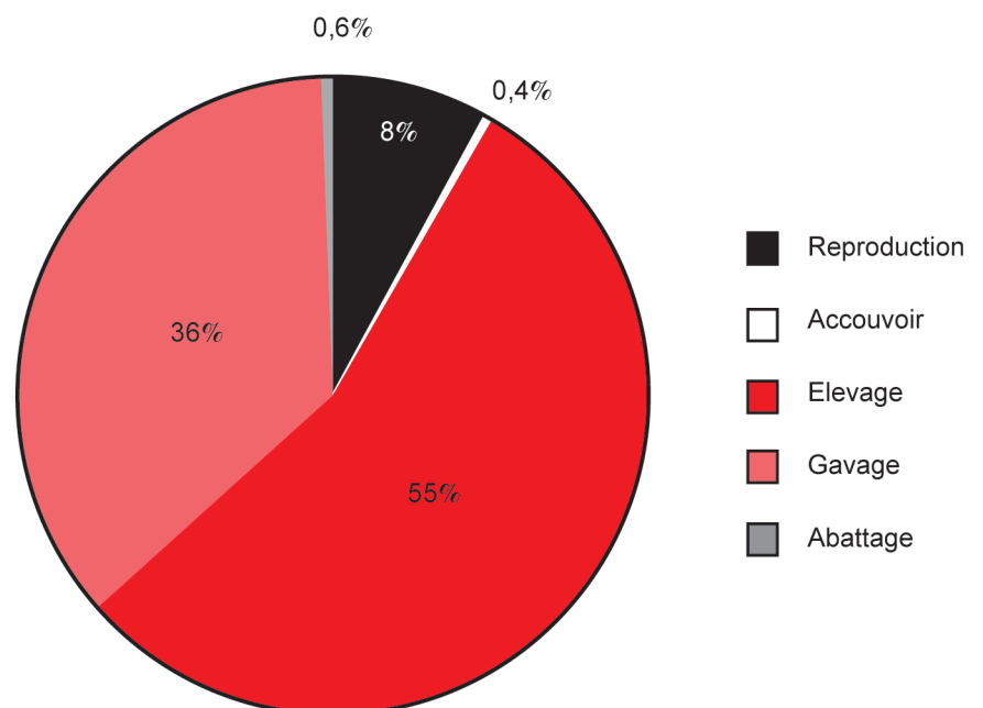
Figure 4. Contribution des différentes étapes du processus de production au potentiel de réchauffement climatique induit par la production de foie gras d'oie (adapté de Arroyo et al 2013f).
