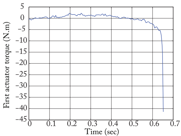
(a) Actuator 1
