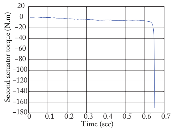
(b) Actuator 2
