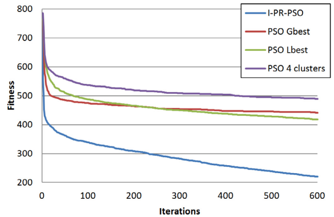
Fig. 13. Rastrigin.
