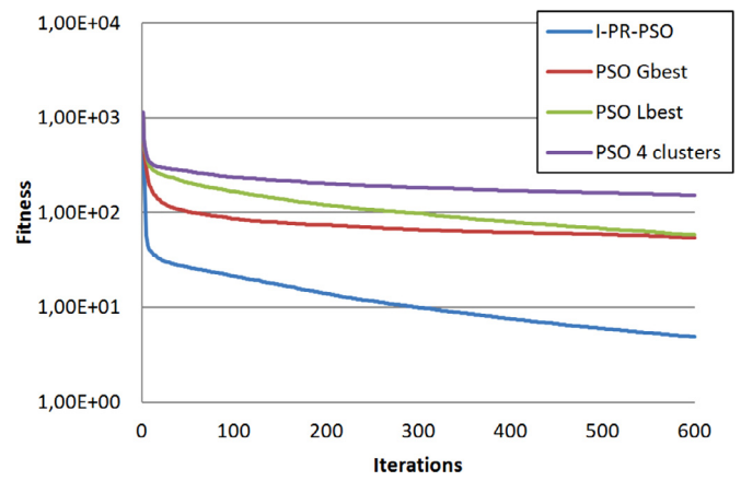
Fig. 12. Griewank.
