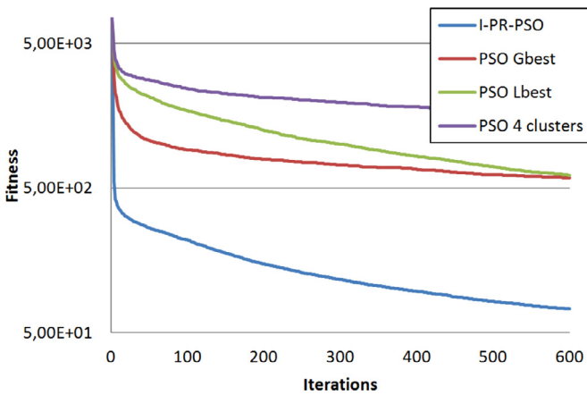
Fig. 21. Bohachevsky.
