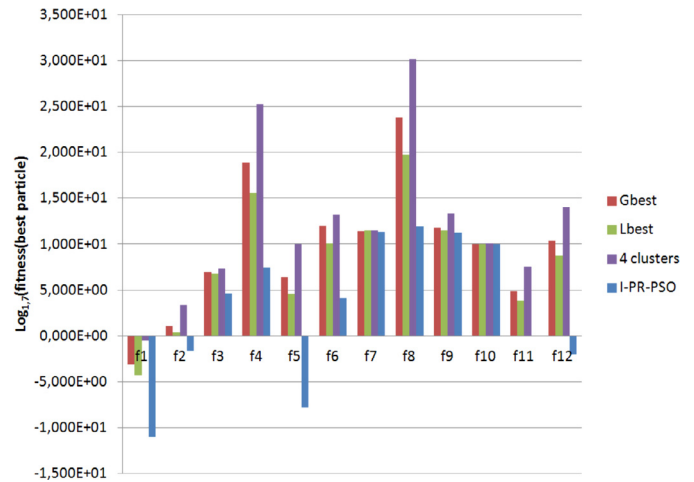
Fig. 7. Dimension 10.
